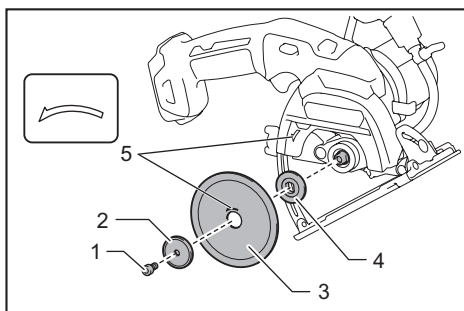
► 1. Perno hexagonal 2. Brida exterior 3. Rueda de diamante 4. Brida interior 5. Flecha
